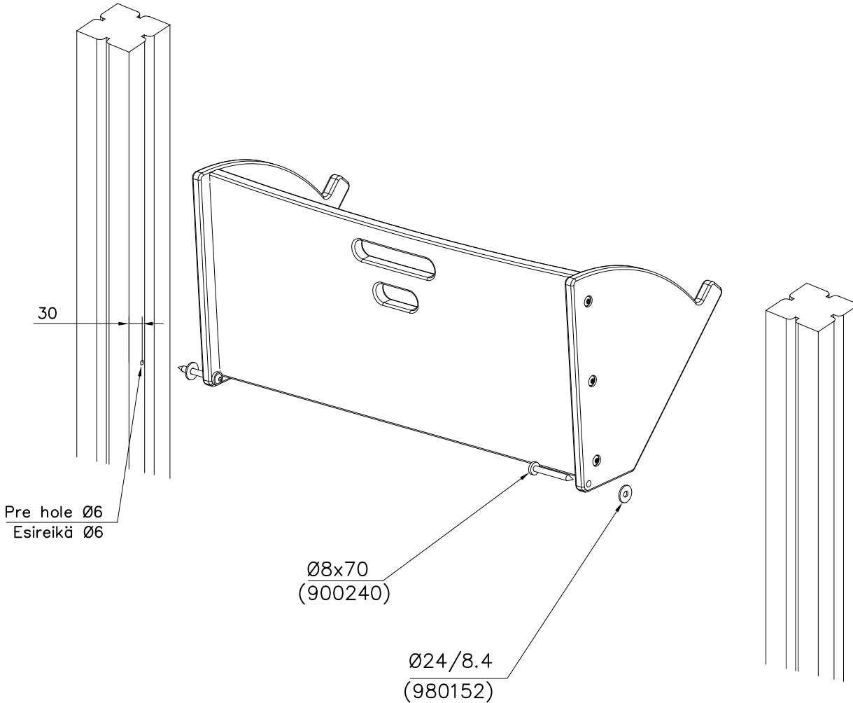
DET 2
