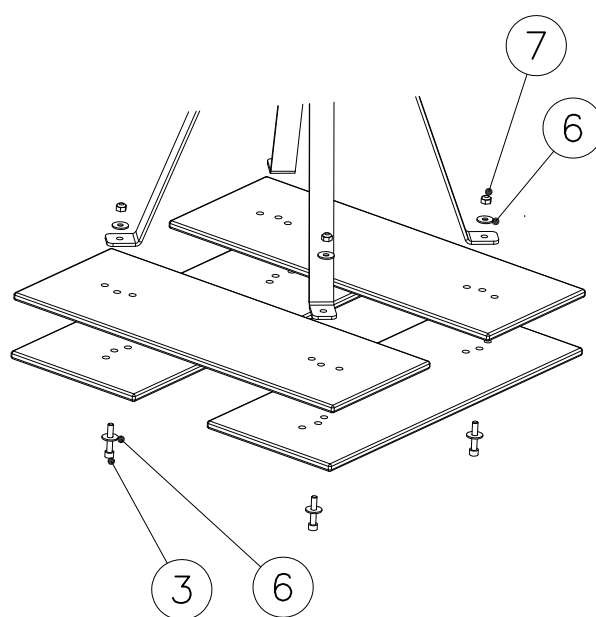
DET 2
