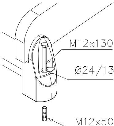
DET 59
