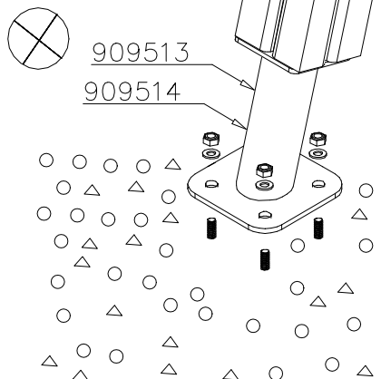
DET 55
