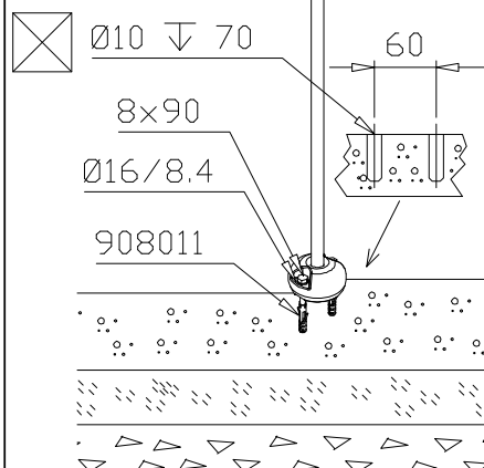
DET 60
