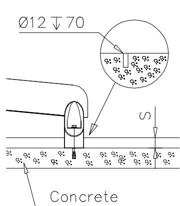
DET 58
