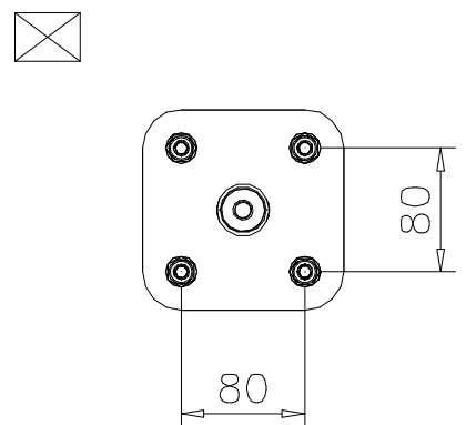
DET 55
