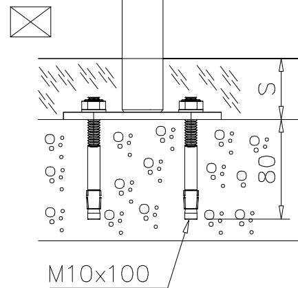
DET 57
