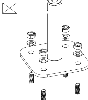
DET 59
