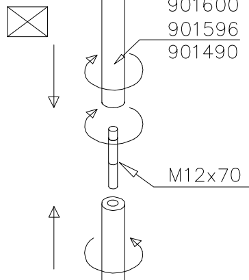
DET 56
