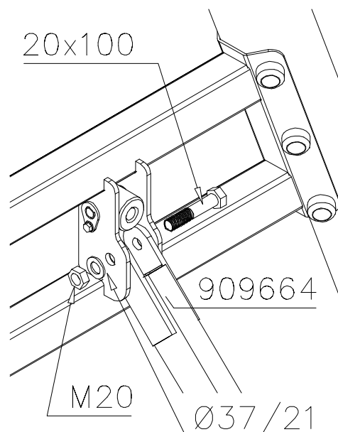
DET 5
