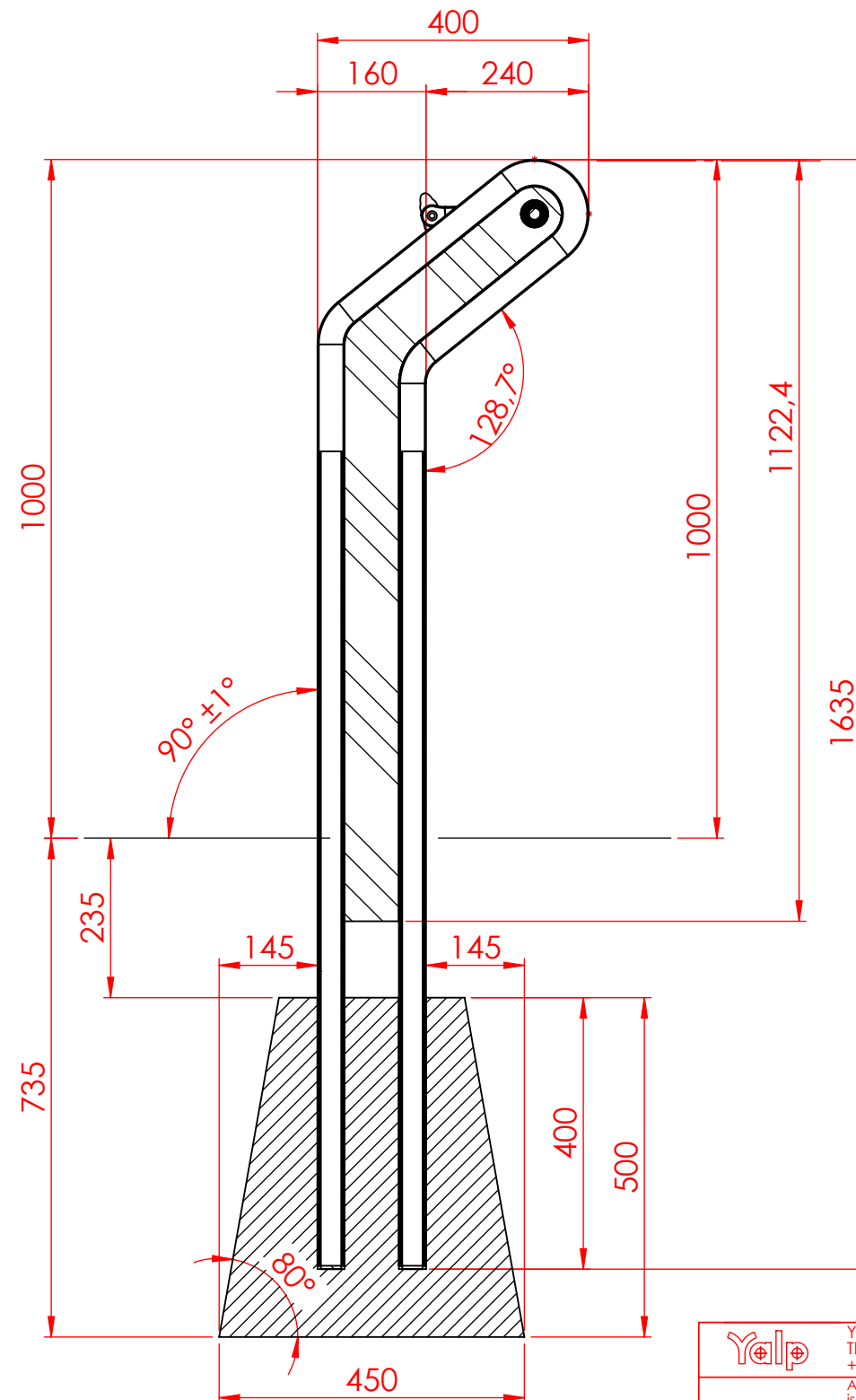
SECTION A-A
