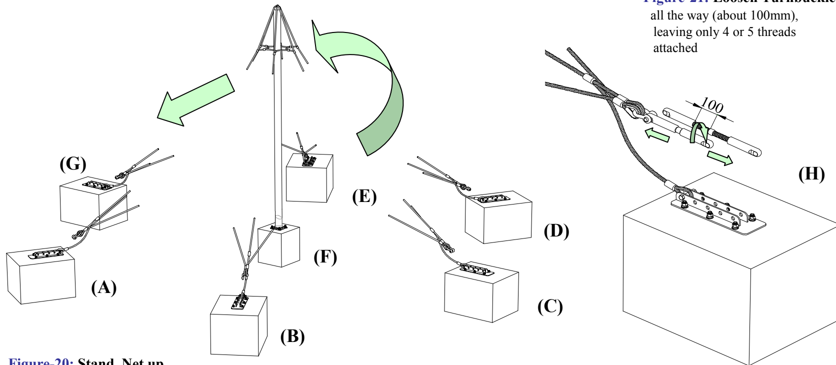
Figure-20: Stand Net up
