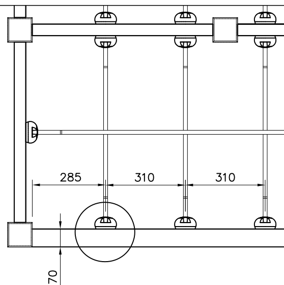
DET 3
