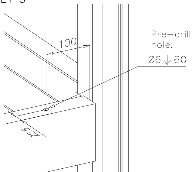
DET 3
